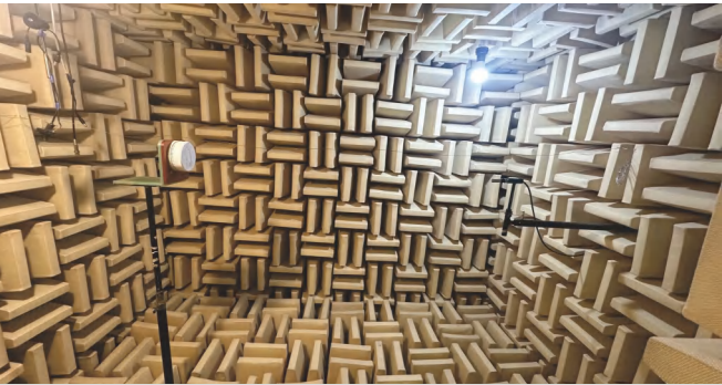
声压测试
